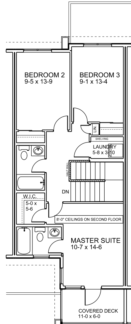
SECOND: 801 SQ FT
